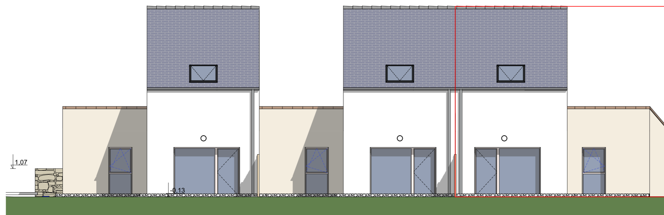
ELEVATION SUD
